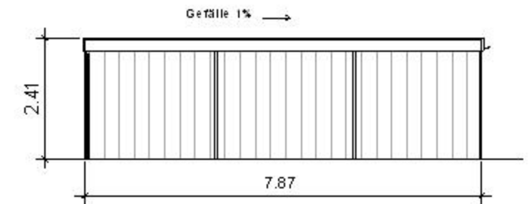
LÄNGSSCHNITT
