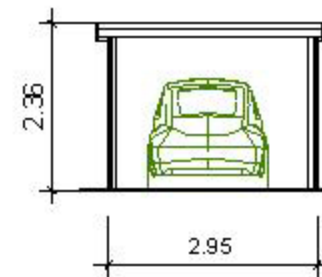
QUERSCHNITT
